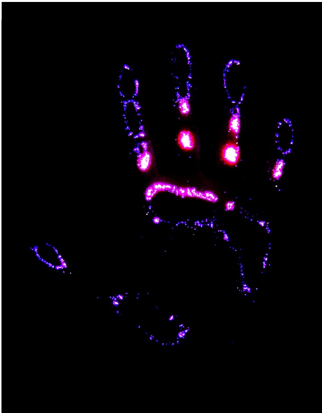
Photo : C4r0 , CC BY-SA 3.0 , via Wikimedia Commons La photographie Kirlian et les travaux de Wilhelm Reich ont déjà mis en évidence l'existence des plans éthériques de la matière.
